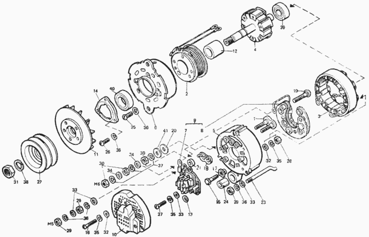
Рис. 47. Генератор 462.3701000
