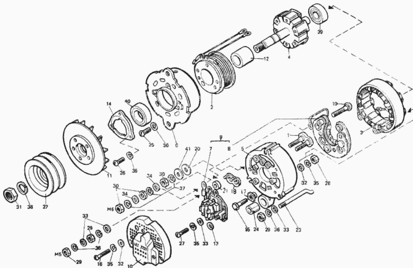
Рис. 47. Генератор 462.3701000
